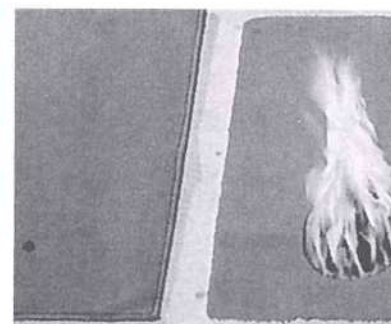
着火1分経過。左側の防災じゅうたんは燃え広がらない
